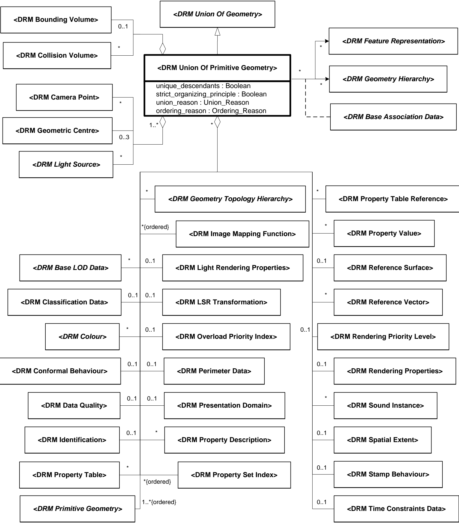
Figure 6.369 — DRM_Union_Of_Primitive_Geometry
